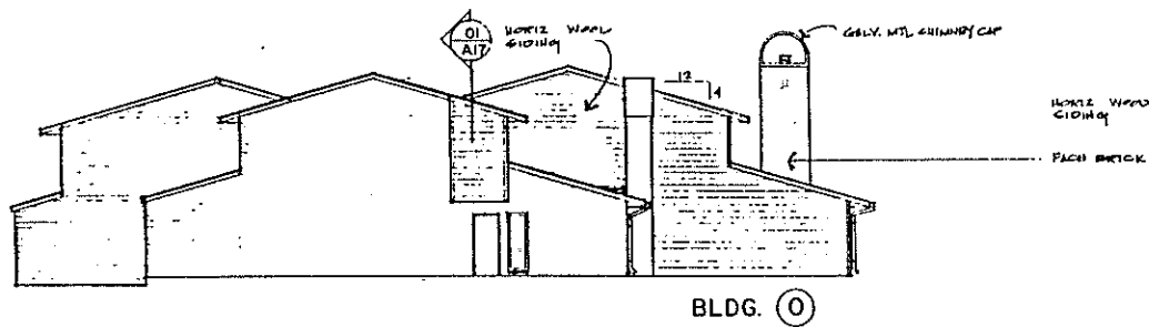
END ELEVATION
