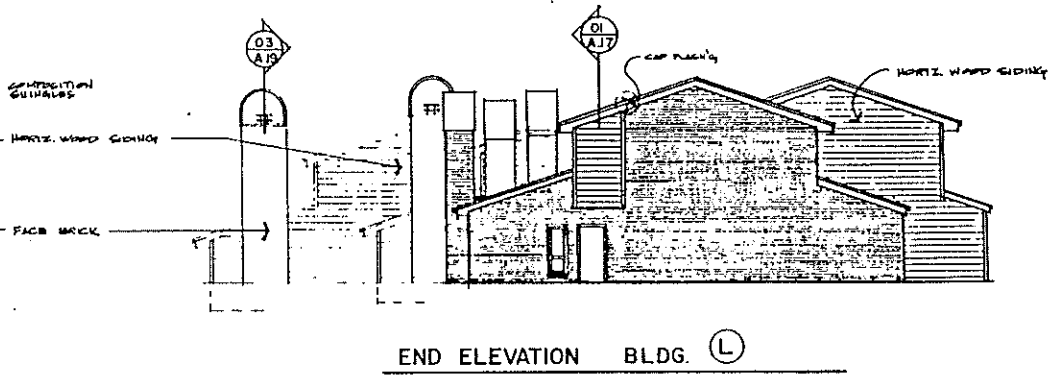
END ELEVATION BLDG. (L)
